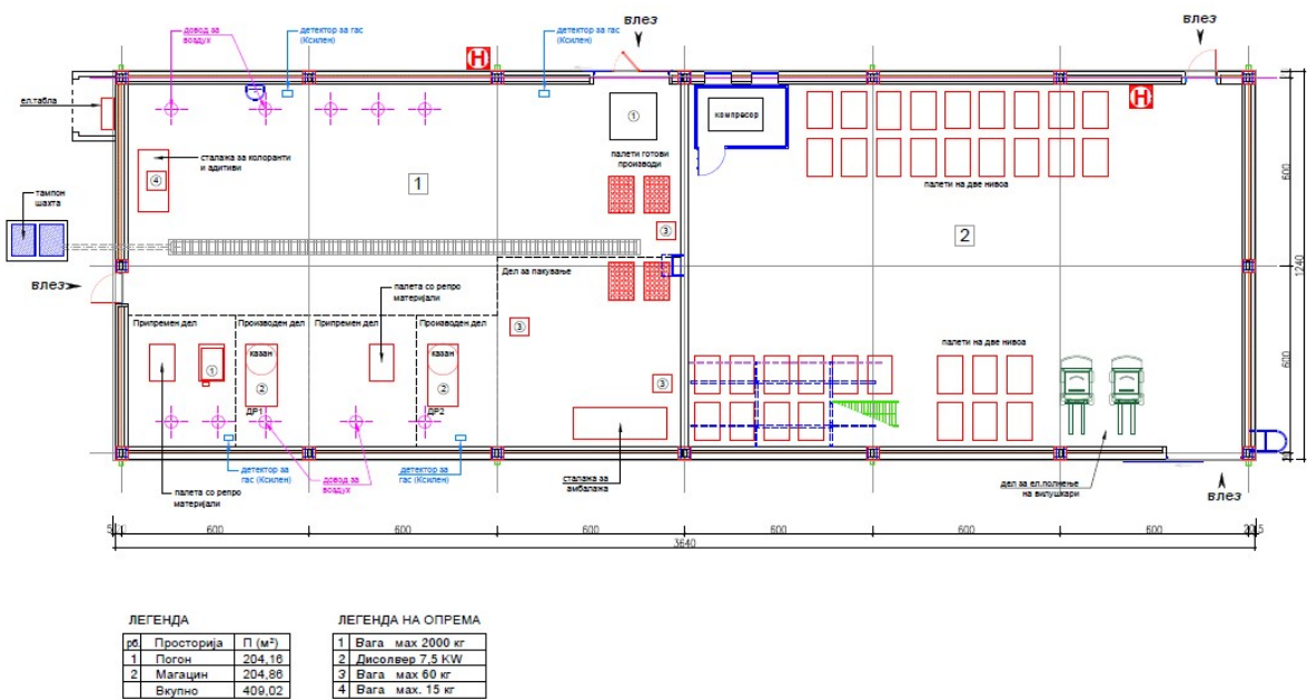
ТЕХНОЛОШКА ШЕМА
