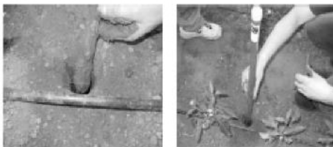
Поставување на тензиометарна постојано место (на поле)
