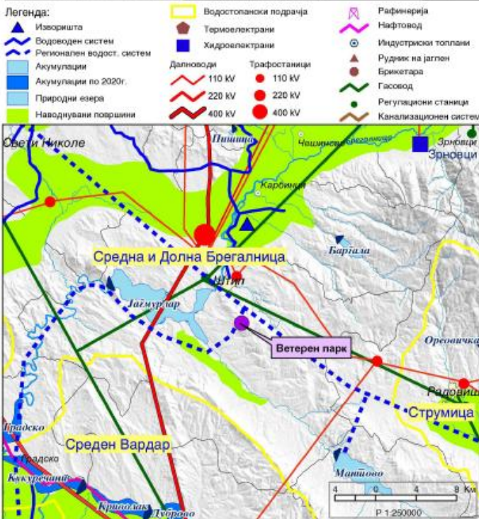
Слика 13. Водостопански подрачја во планскиот опфат (извор: Просторен план на РМ) Низ дел од просторот поминува планиран регионален водоснабдителен систем Црна Река.
