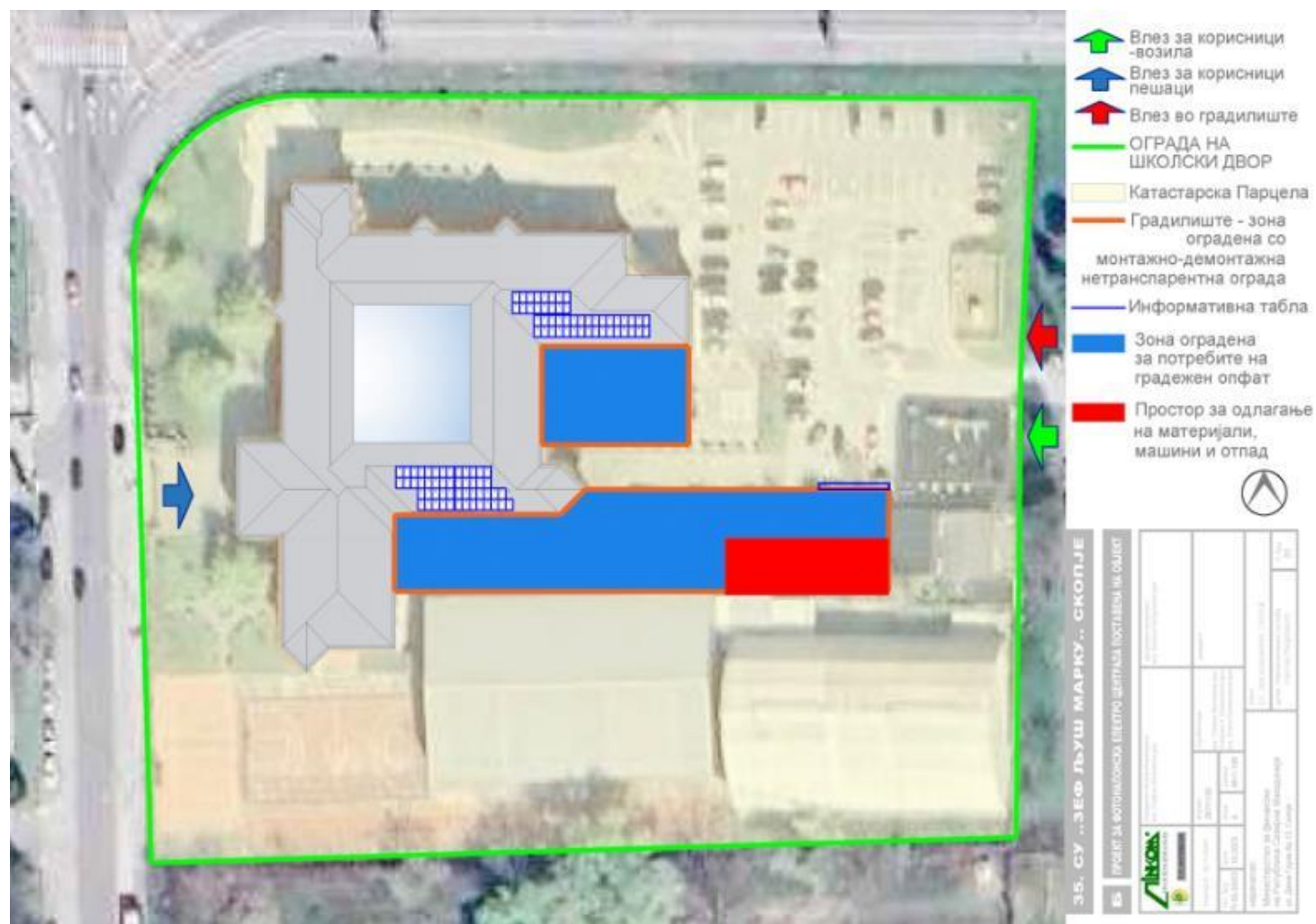
Слика: Индикативна шема на градилиште (шематски приказ)
