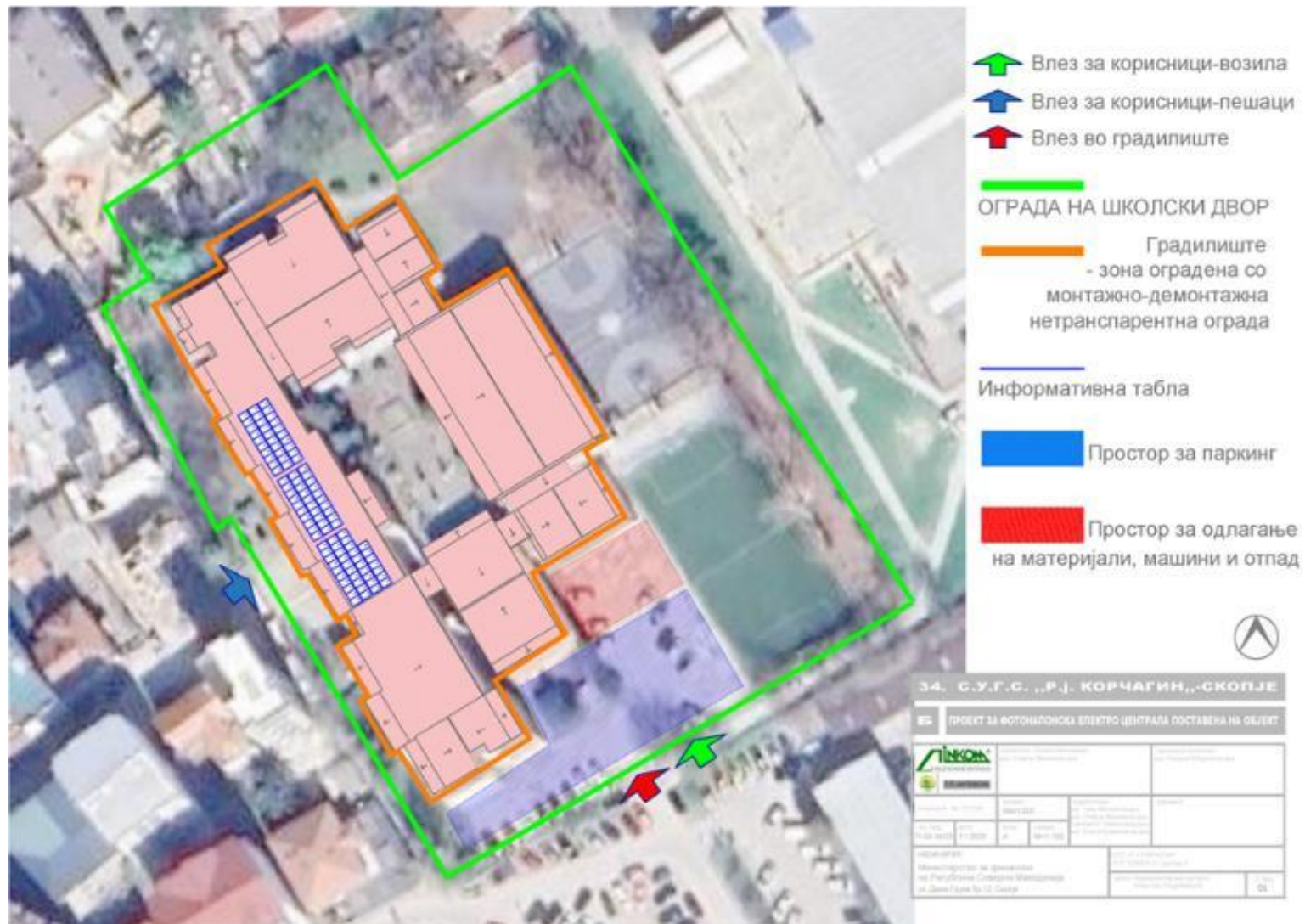
Слика: Индикативна шема на градилиште (шематски приказ)
