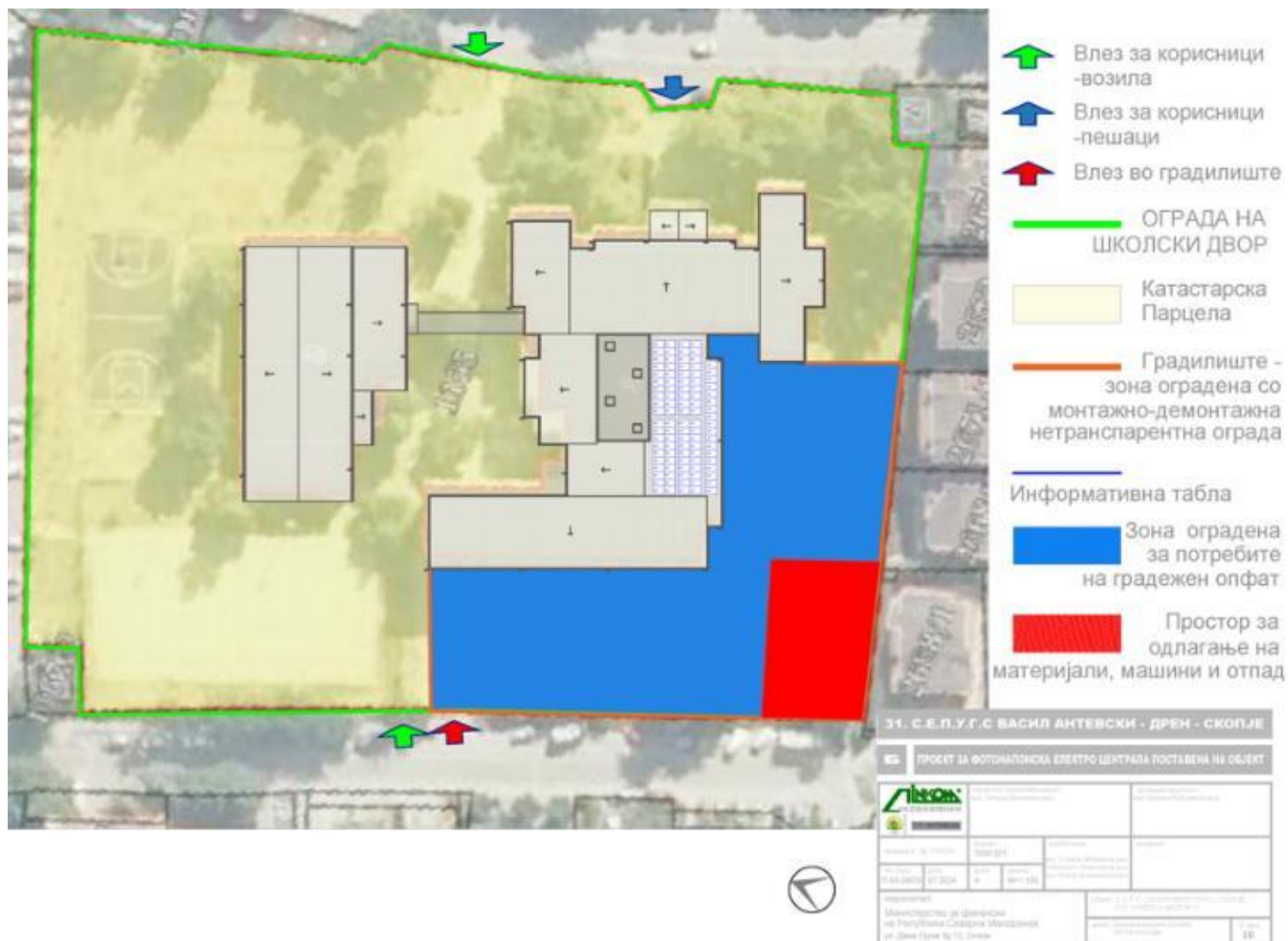
Слика: Индикативна шема на градилиште (шематски приказ)
