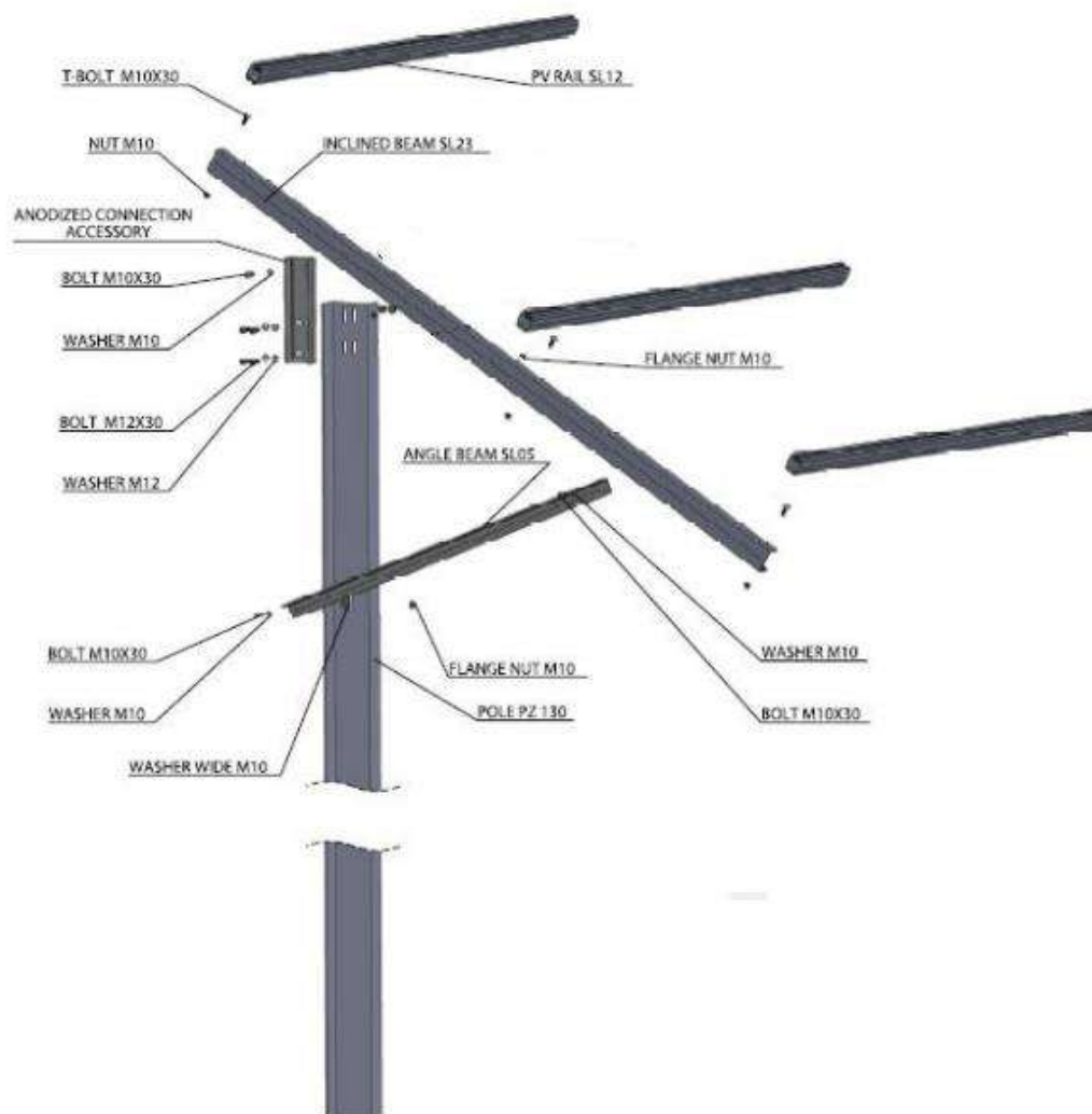
Слика 11. Приказ на целата монтажна конструкција
